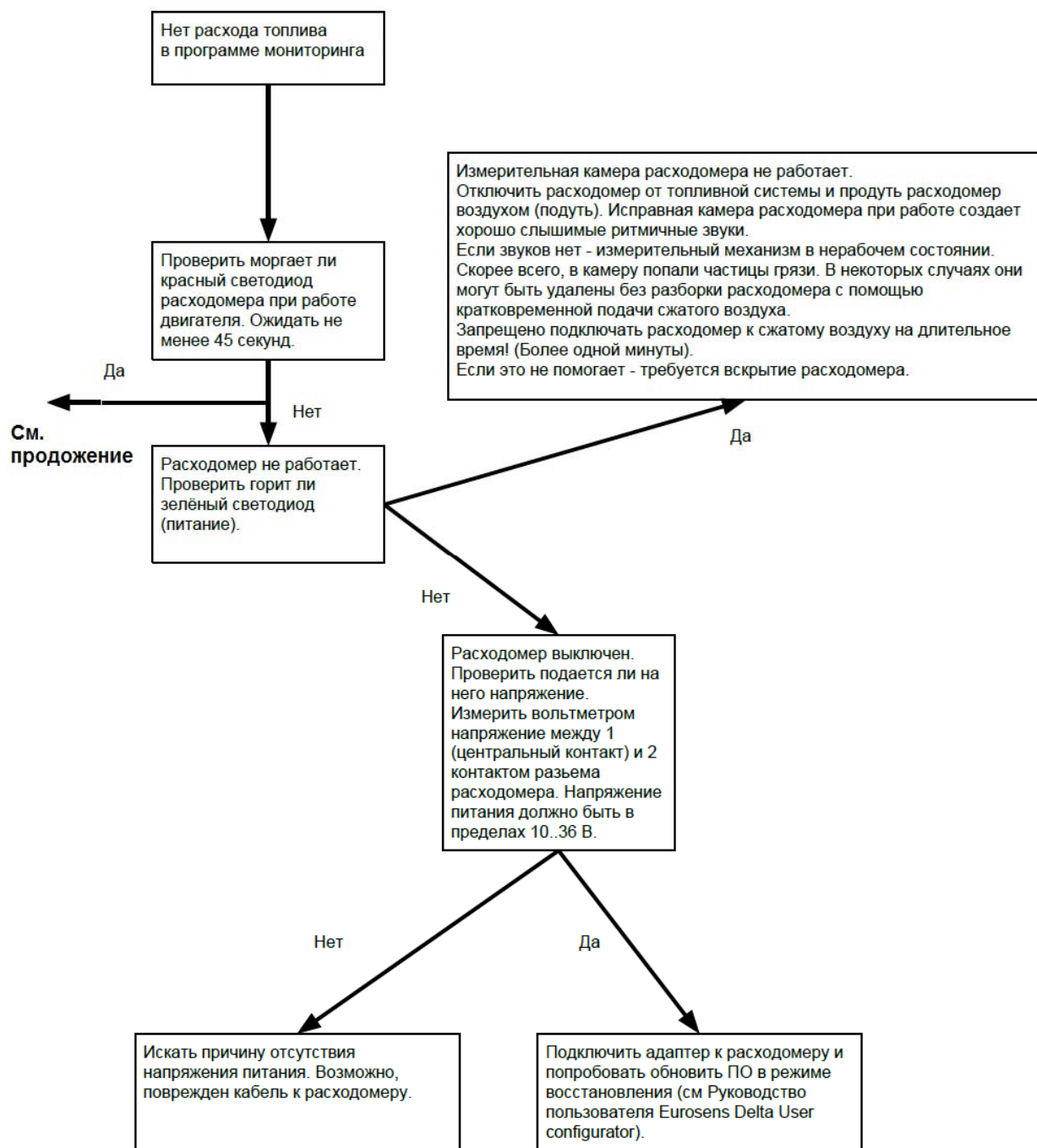
Рис.11. Экспресс-диагностика датчиков расхода EUROSENS Direct (Начало)
