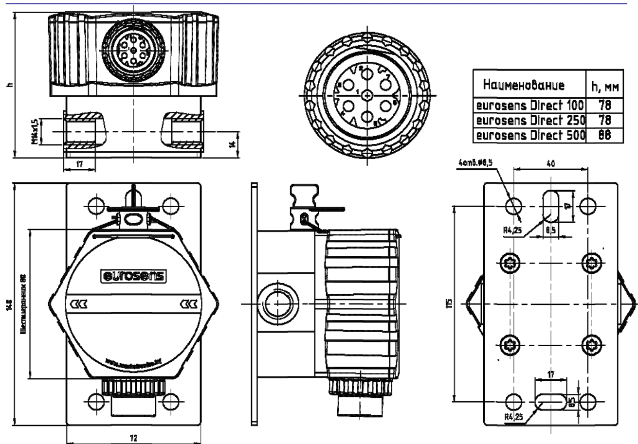
Рис.15. Габаритные и установочные размеры EUROSENS Direct
