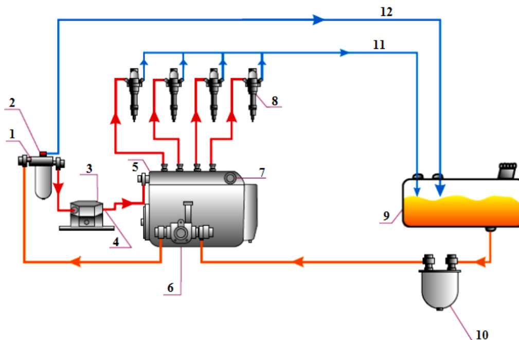
Рис.4. Схема установки датчика Direct «На давление»
