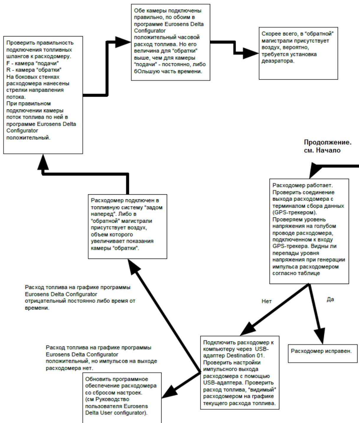
Рис.14. Экспресс-диагностика датчиков расхода EUROSENS Delta (Продолжение).
