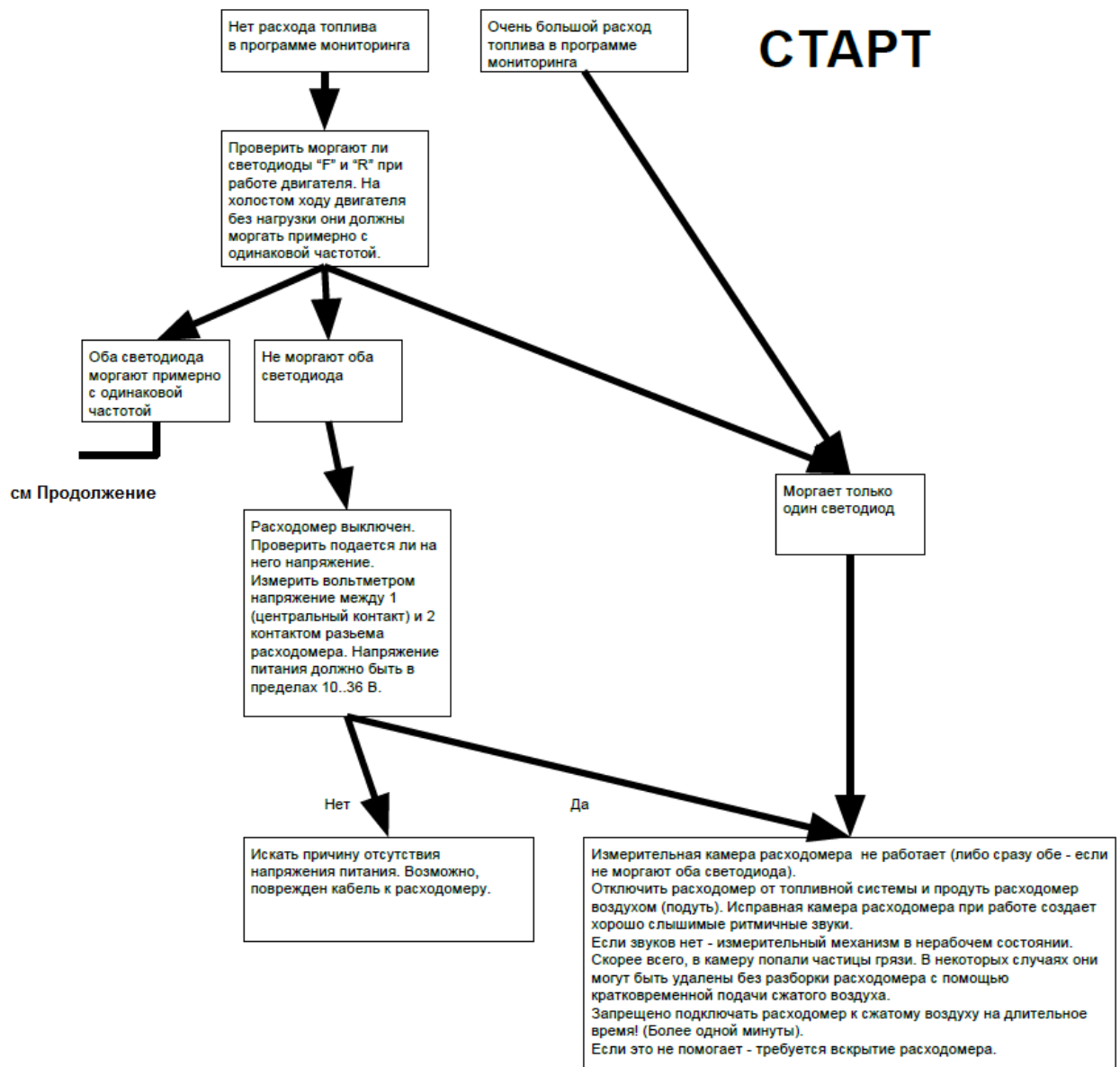
Рис.13. Экспресс-диагностика датчиков расхода EUROSENS Delta (Начало)
